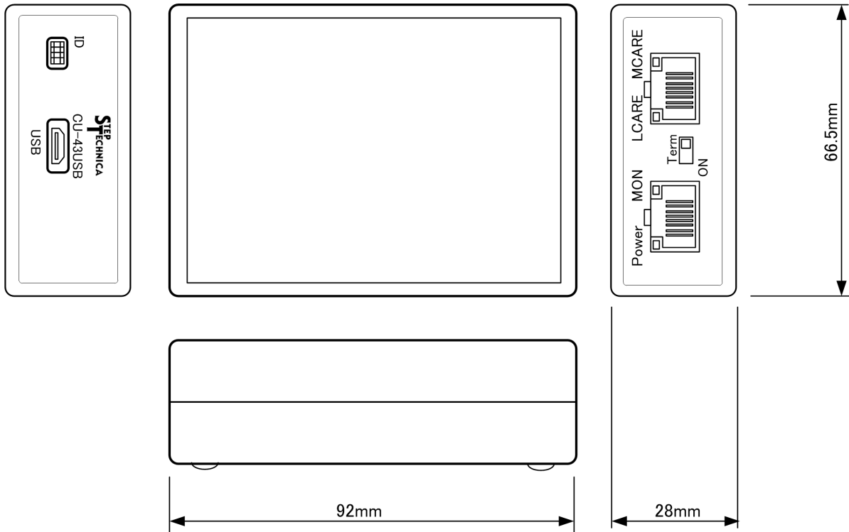
図 4-2 外形寸法図
