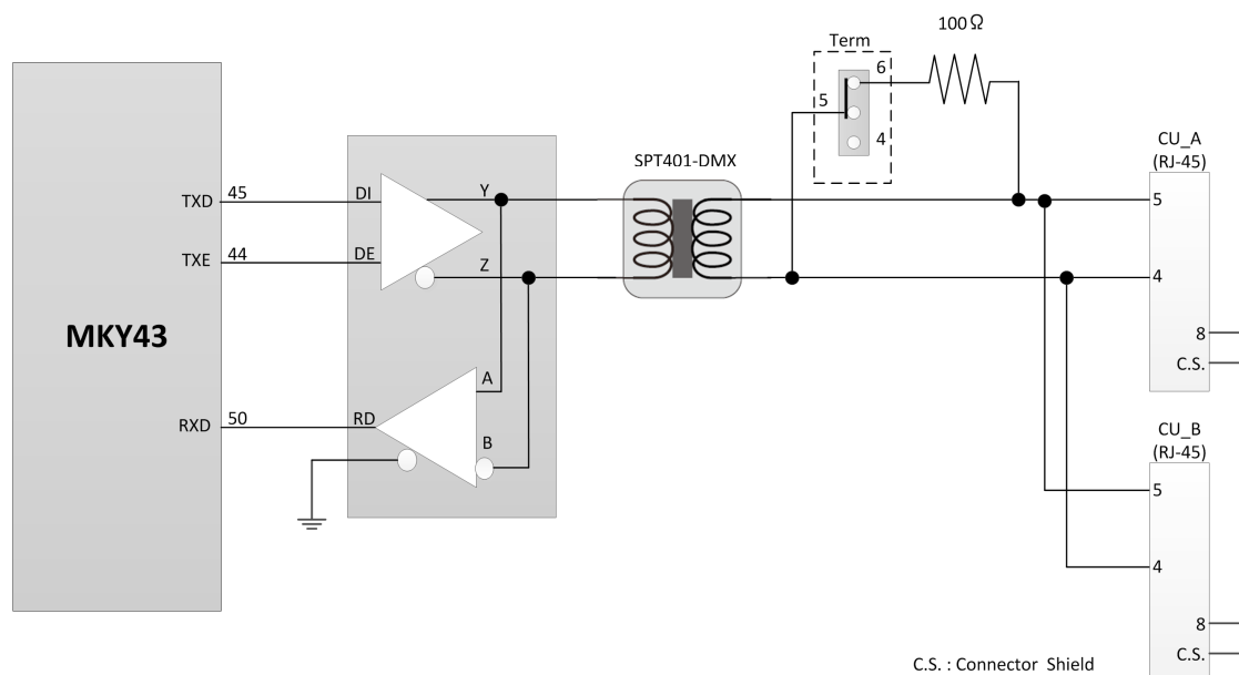
図 4-1 CUnet 接続図
